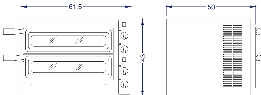
Vista Elevación
